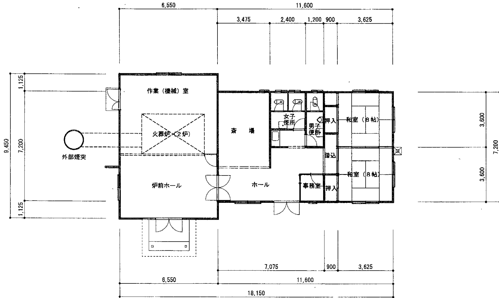
解体建物平面図
