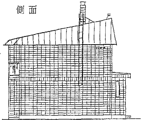
側 面 図
