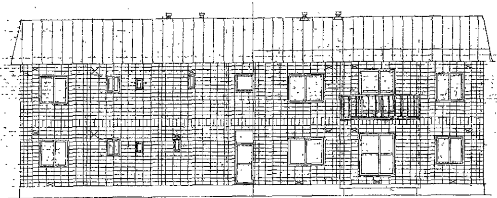
(北 面)
