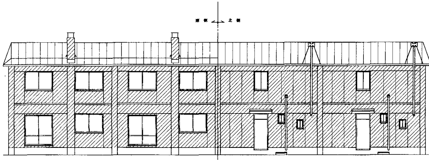
南側立面図
