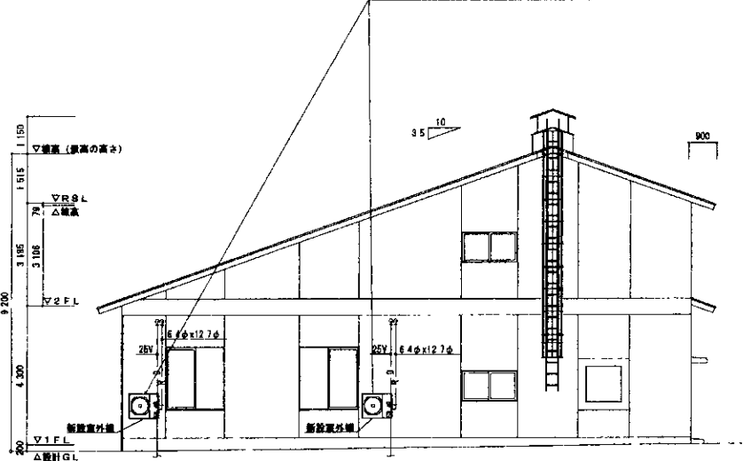
北葺立面図 S=1/100
