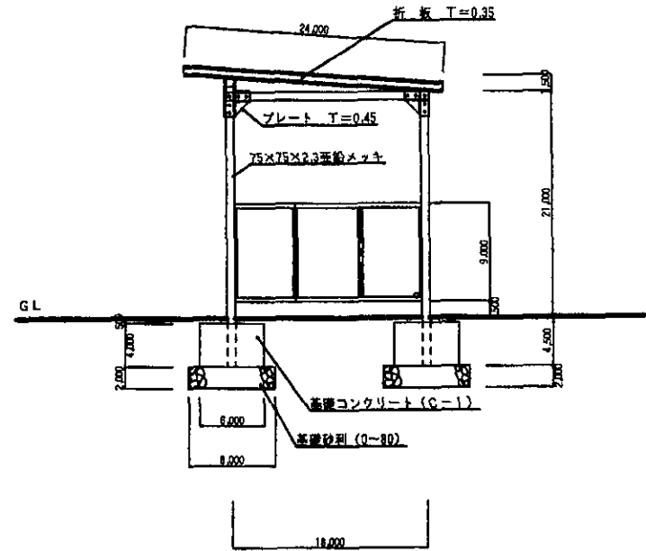
自転車置場断面図
