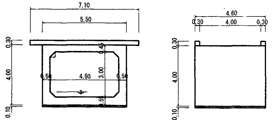
断面図
