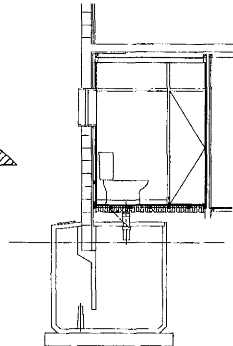
改修後詳細図
