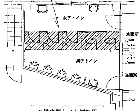
2階東側トイレ詳細図
