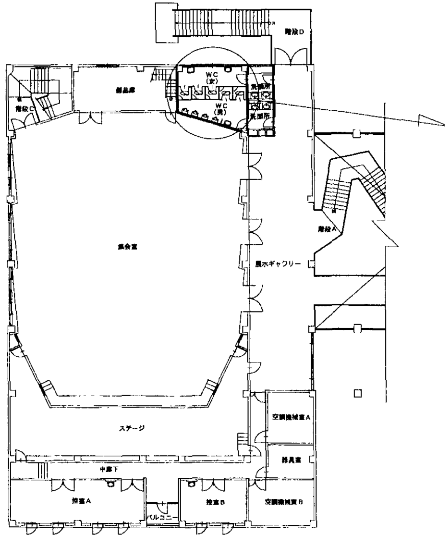
2階平面図
