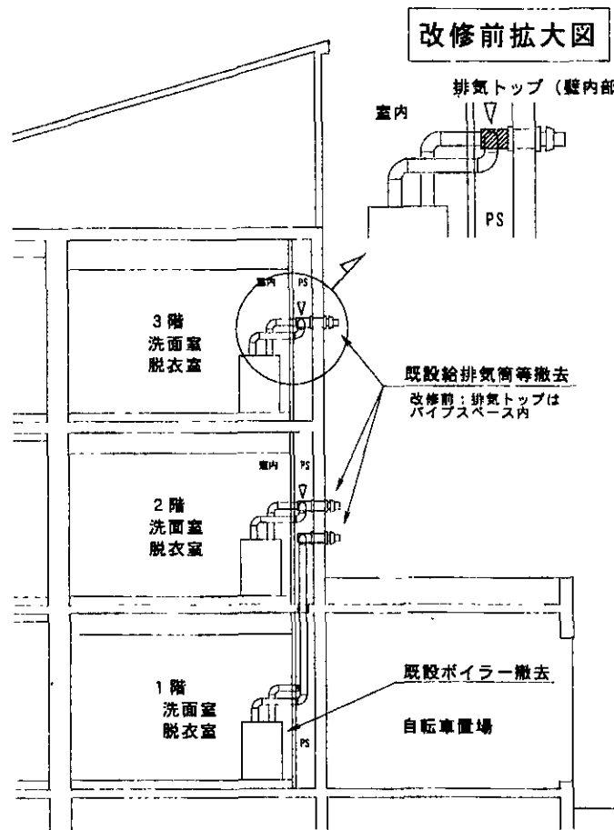
改修前詳細図
