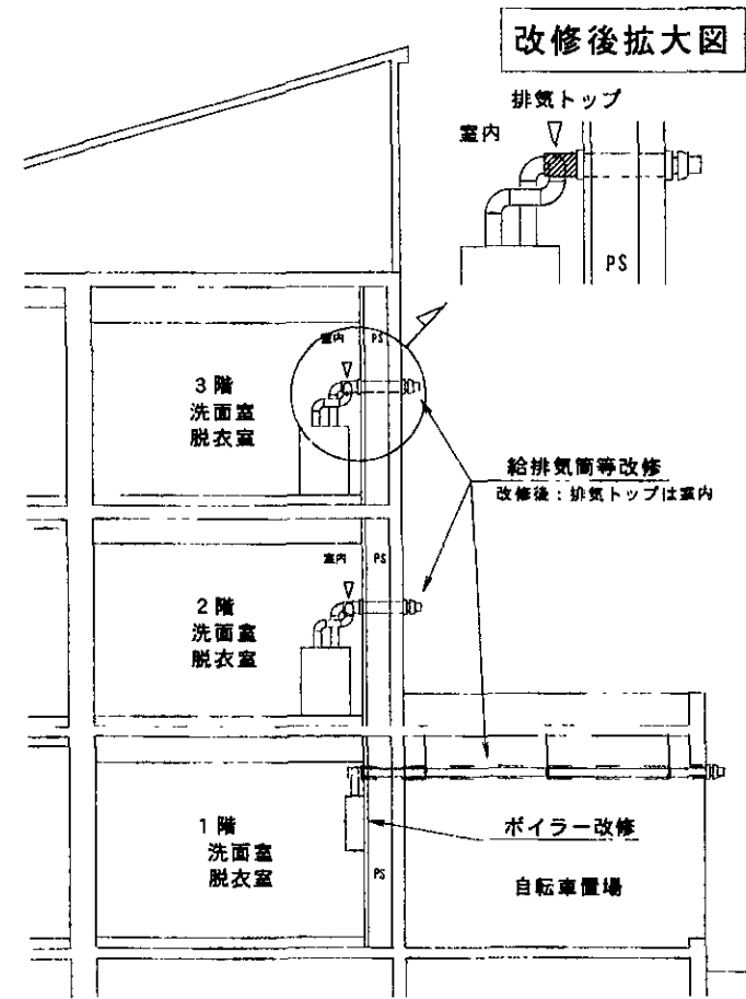
改修後詳細図
