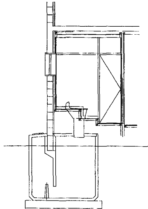
改修前詳細図
