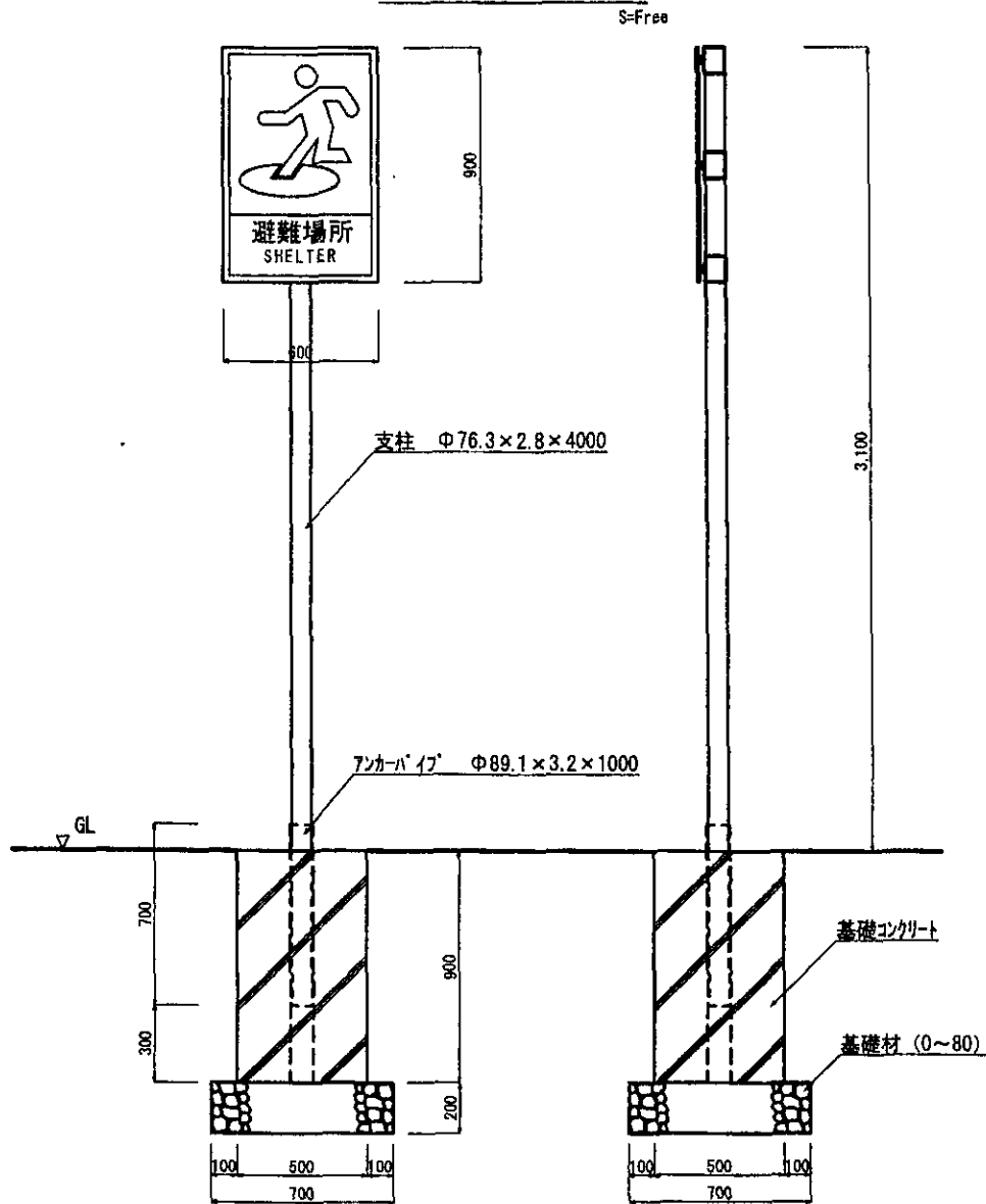
姿 図
