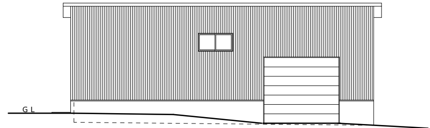
南側立面図
