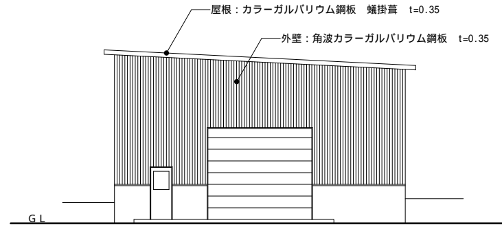
東側立面図
