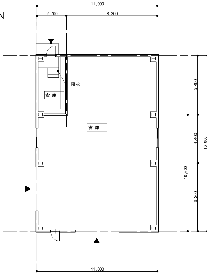
平面図
