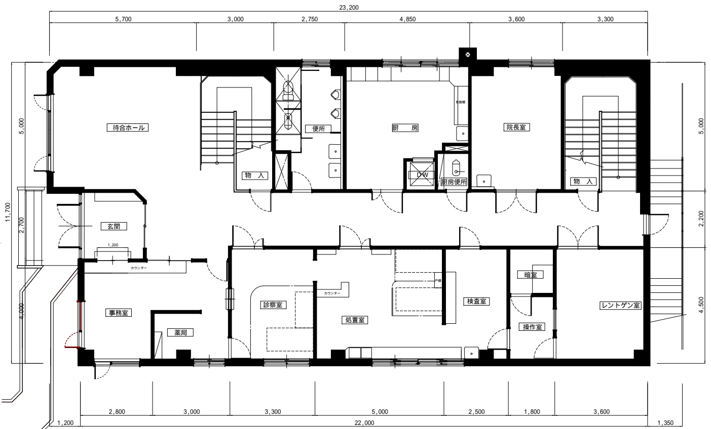
1階平面図 (改修前)
